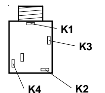
die Anschlüsse der Kopfhörerbuchse (K)
